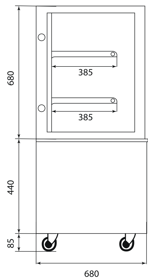
Vista Lateral
