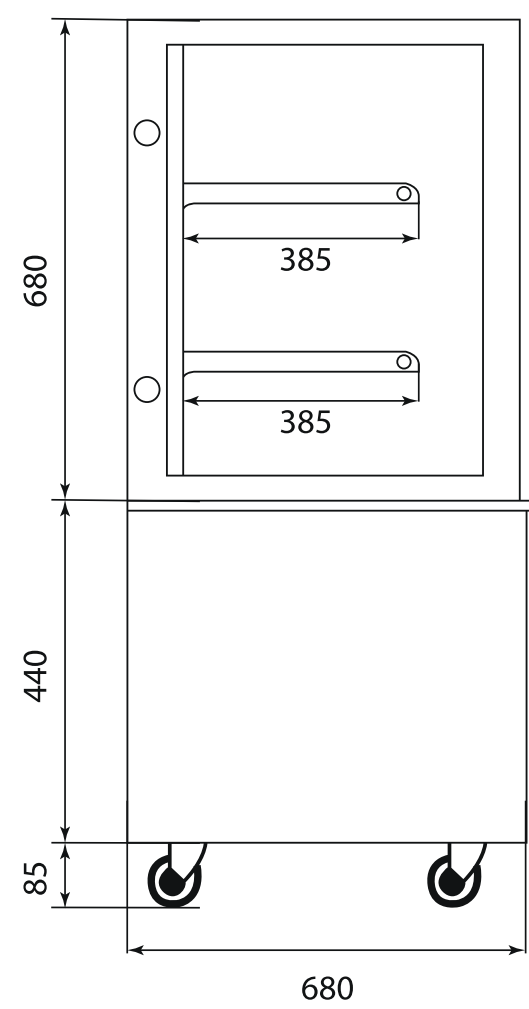
Vista Lateral
