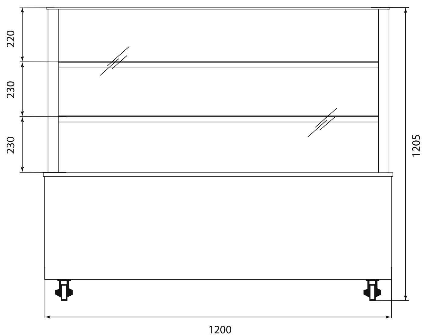
Vista Frente
