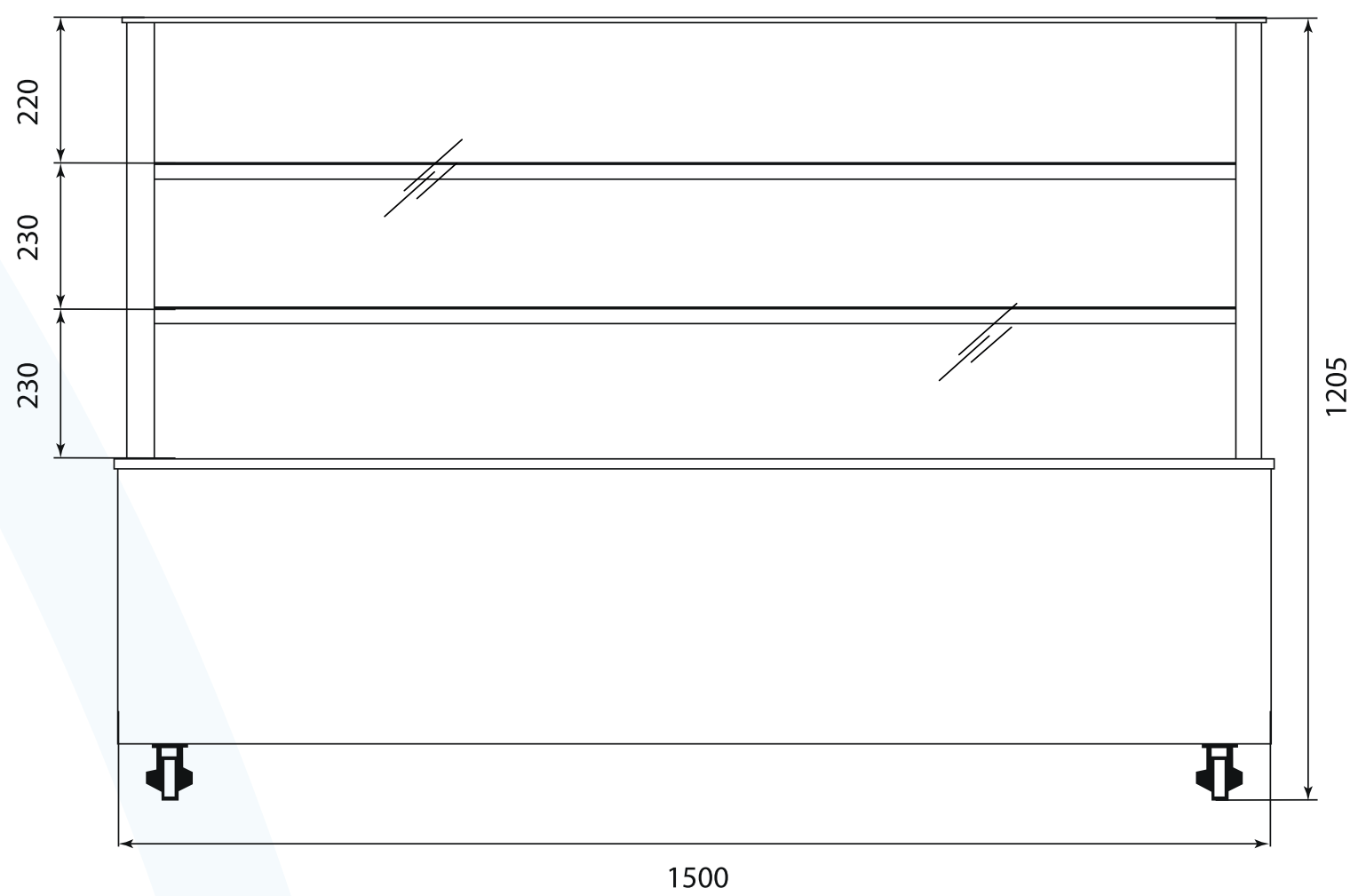
Vista Frente
